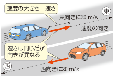
↑速さと速度
